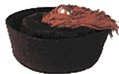
清代朝冠帽
